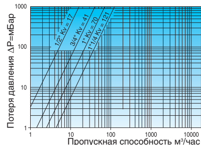
Диаграмма потери давления (испытано водой)
