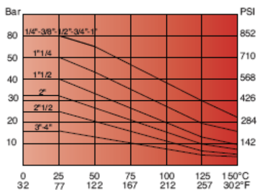
Диаграмма давление/температура
