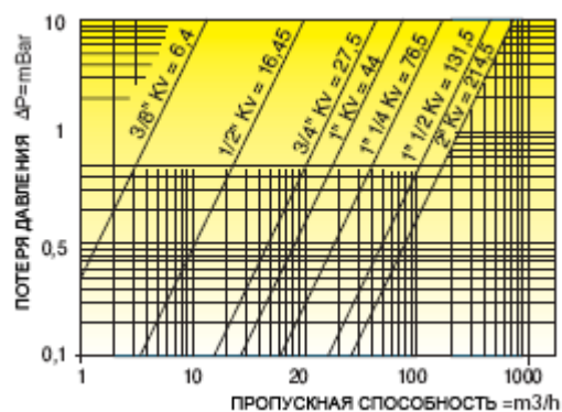
Диаграмма потери давления
