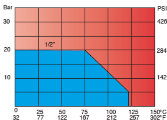
Диаграмма давление/температура
