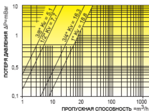
Диаграмма потери давления (Тестирован с воздухом)
