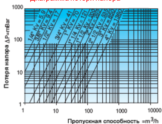
Диаграмма потеря напора
