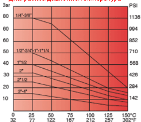
Диаграмма давление/температура
